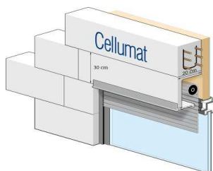
U-Lateien
