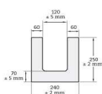
U-blokken
